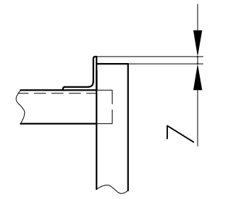
Вуз Γ (1:5)
