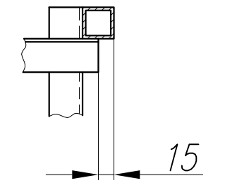
В-В (1:5)
